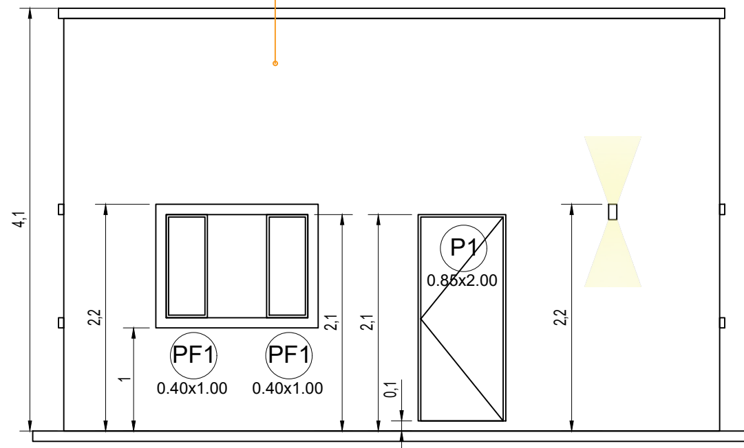
VISTA - C
