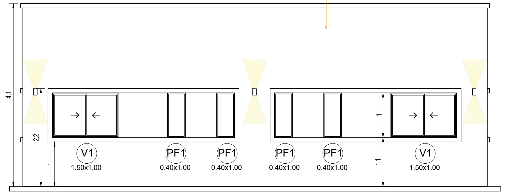
VISTA - D
