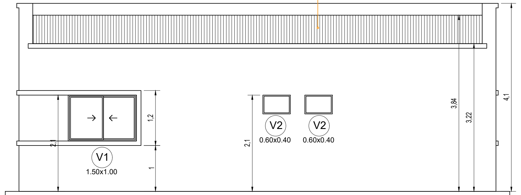
VISTA - B
