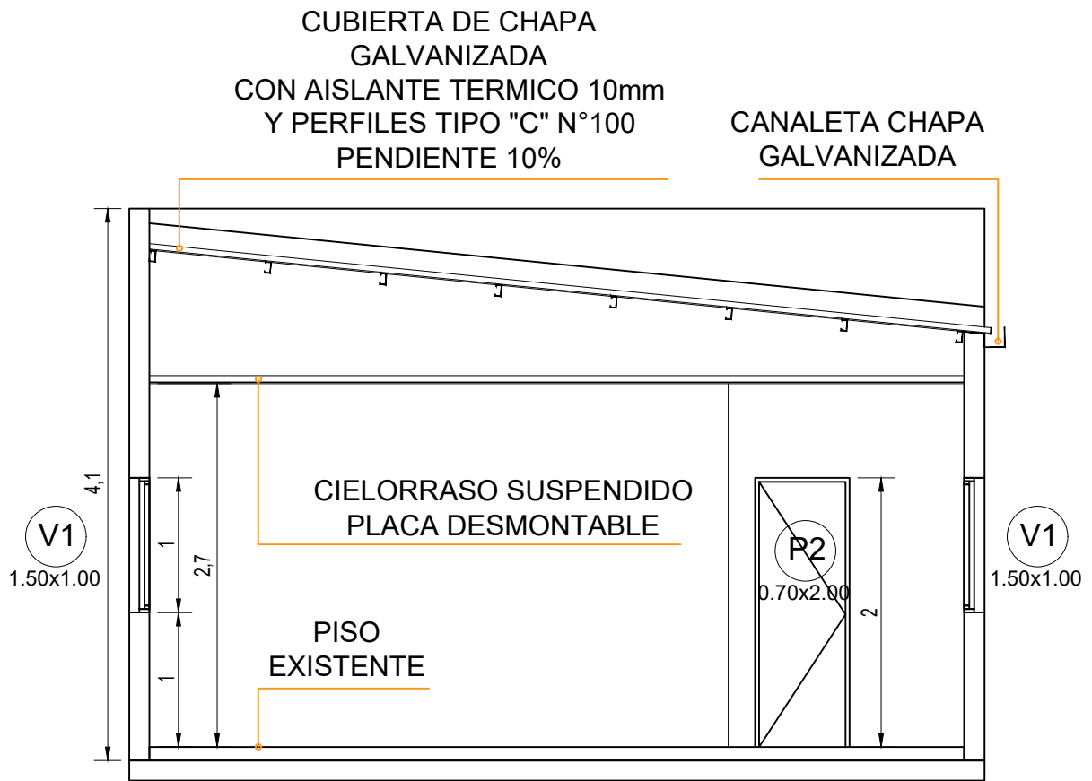
CORTE A-A
