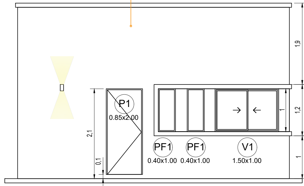
VISTA - A
