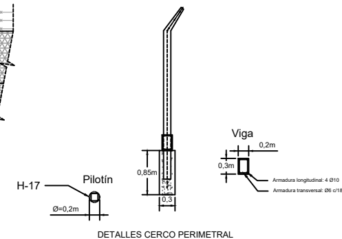
DETALLES CERCO PERIMETRAL
