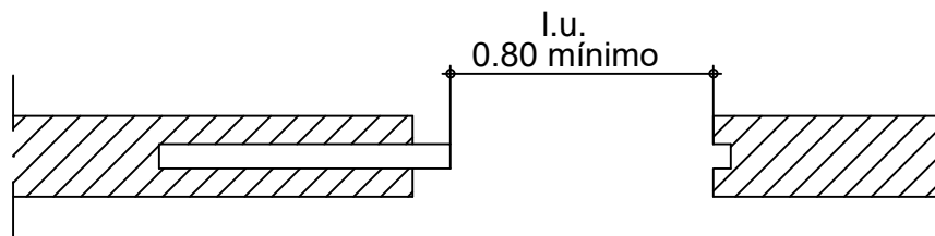
3. Hoja corrediza
