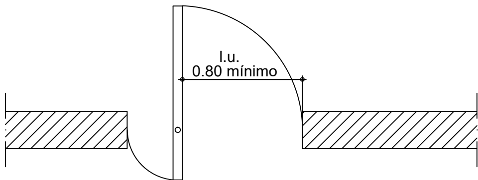
2. Hoja pivotante
