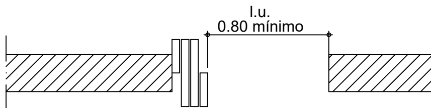
4. Hoja plegadiza
